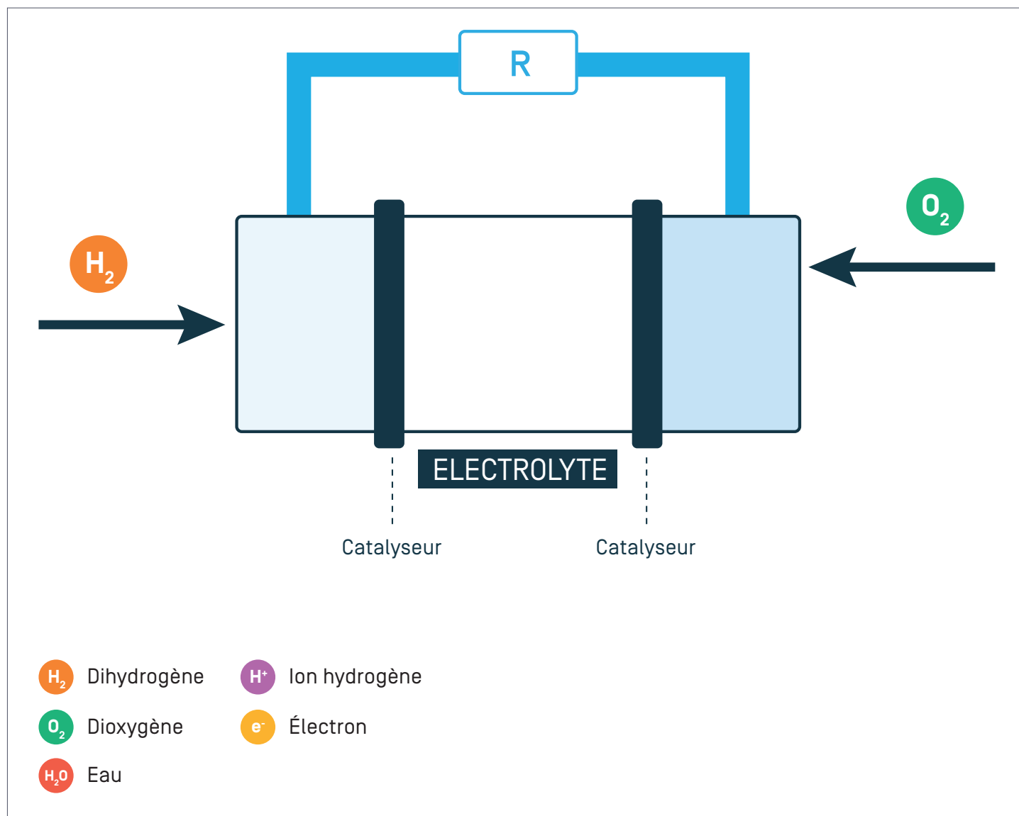
Schéma de la pile à combustible.
