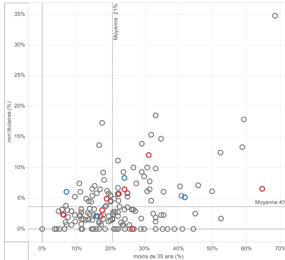
Taux d'enseignants non titulaires en fonction du taux d'enseignants âgés de moins de 35 ans POITIERS - Moyennes par collège public de l'académie
